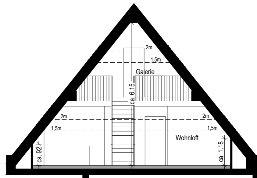
Schnitt 2-2
