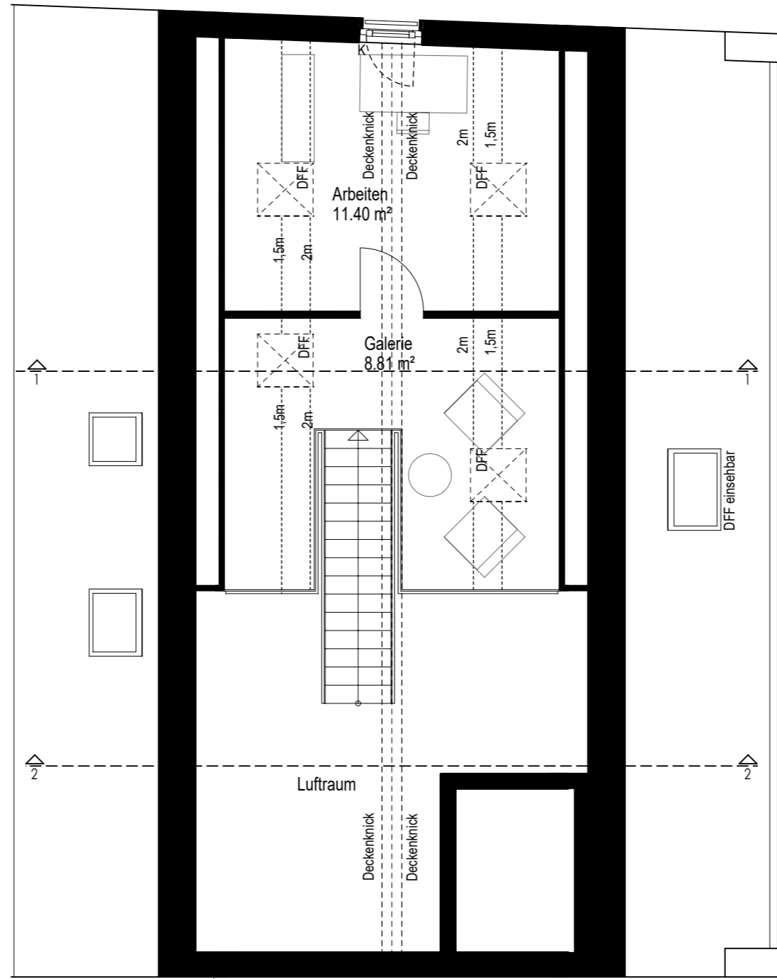
5.OG
