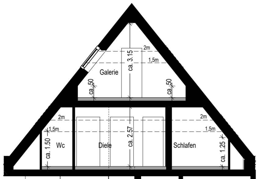
Schnitt 1-1
