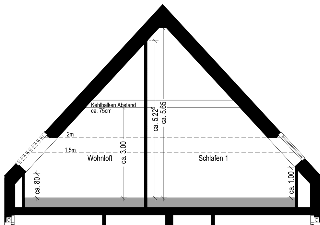
Schnitt 1-1
