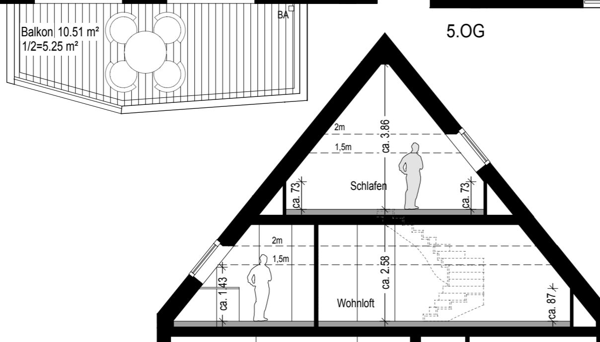
Schnitt 1-1
