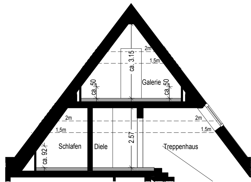
Schnitt 1-1
