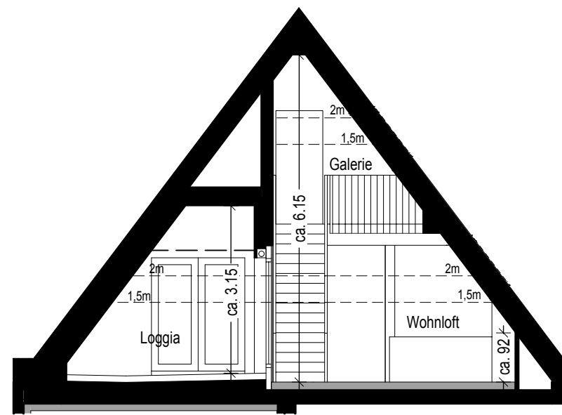
Schnitt 2-2
