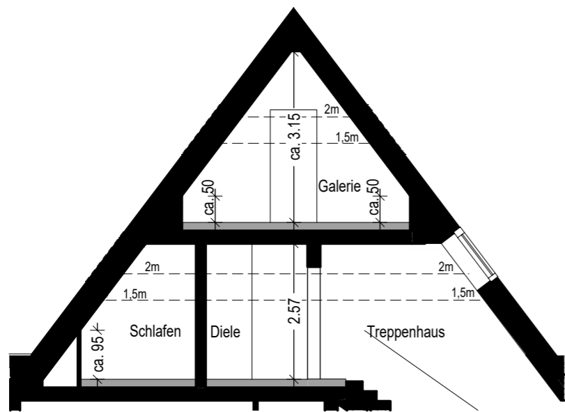
Schnitt 1-1
